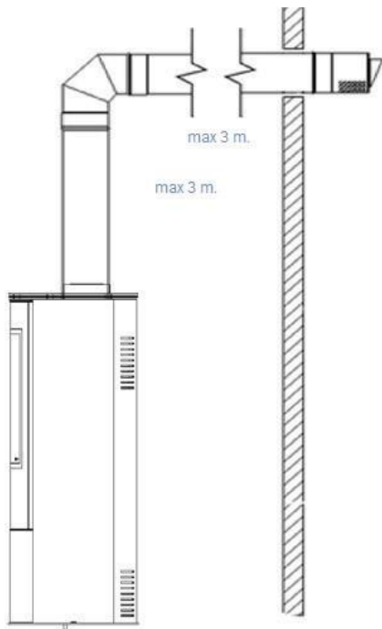
Abb. 5. Führung des konzentrischen Schornsteinsystems
