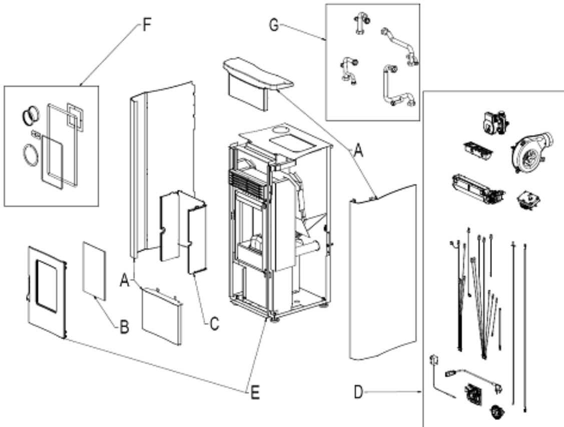
Fig. 1 - Explosionszeichnung
