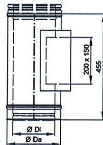
Putztüranschluss (Unterdruck)
