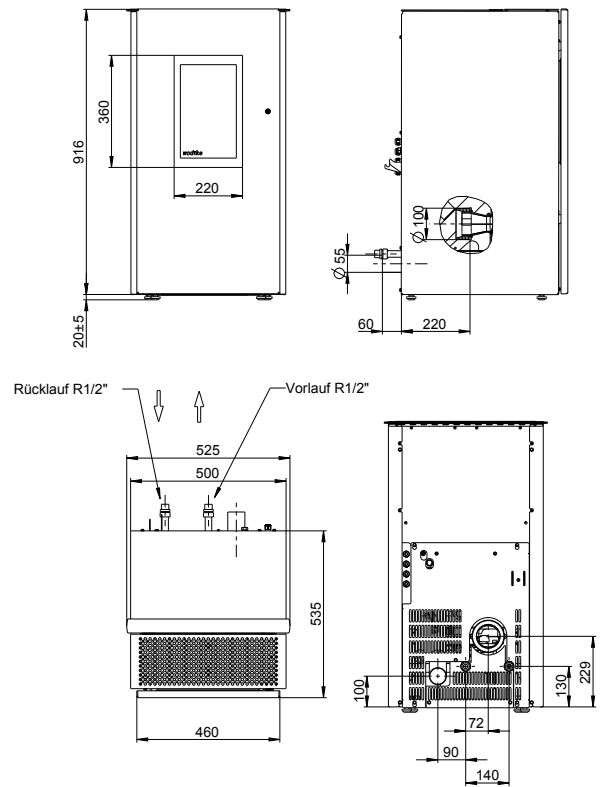
Abb. 103: Maßzeichnung "Pat" Waterplus
