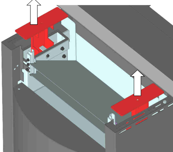
Abb. 62: Entfernen Abdeckung Heizgaszüge
