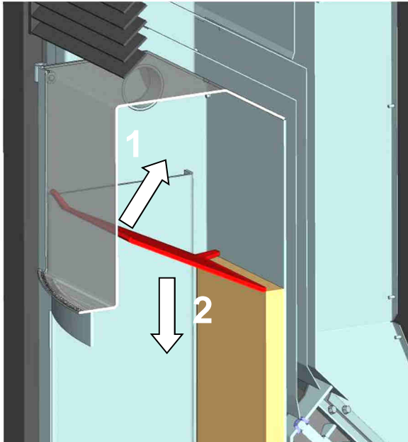
Abb. 57: Entnahme vordere Umlenkplatte
