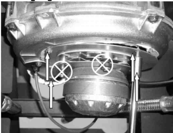
Abb. 86: Demontage Gebläsemotor
