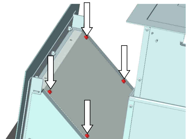
Abb. 40: Demontage Abdeckung PE Nova
