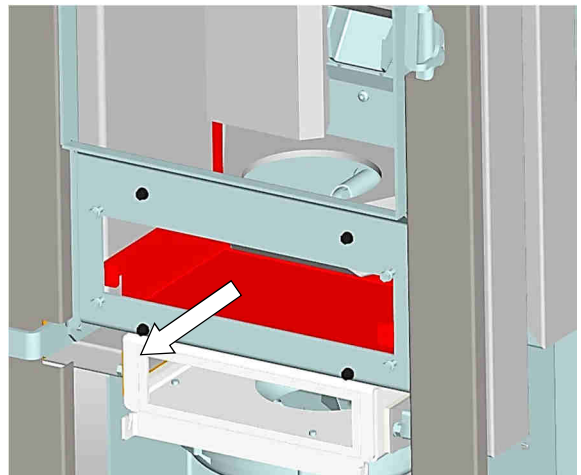
Abb. 54: Entnahme Bodenblech
