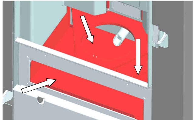
Abb. 81: Reinigung Topfhalter
