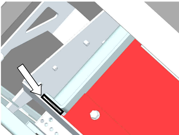
Abb. 74: Soll- Position Dichtschnur links
