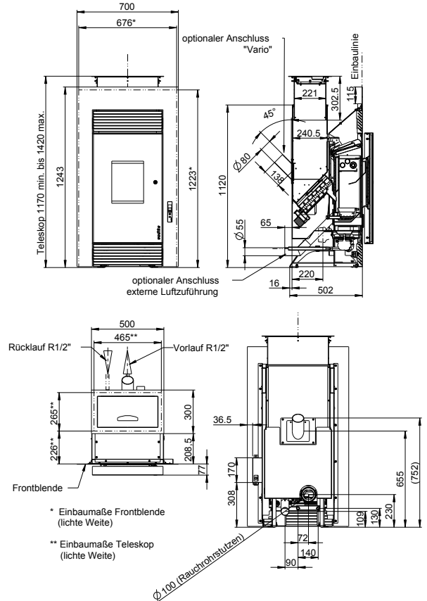
Abb. 105: Maßzeichnung "PE Nova" Waterplus
