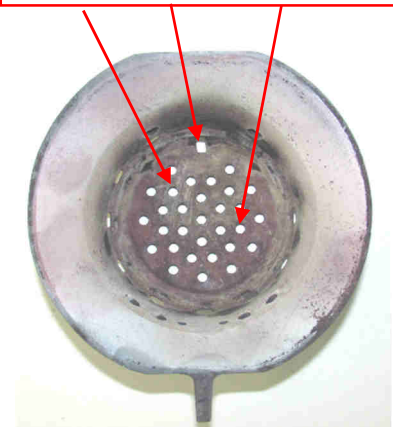
Abb. 35: Brennertopf sauber
