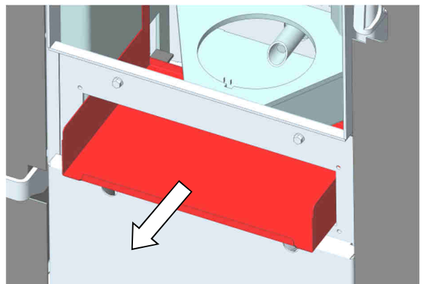
Abb. 82: Entnahme Bodenblech
