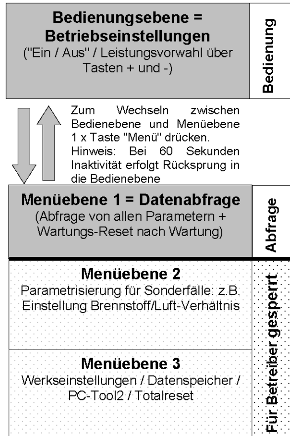
Abb. 6: Bedienebenen
