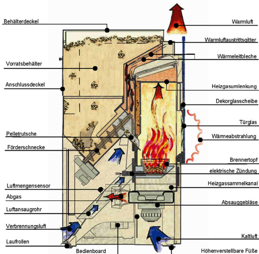
Abb. 3: Funktionsskizze Pelletofen Airplus
