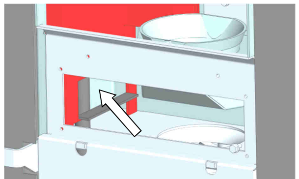
Abb. 83: Reinigung Heizgaszüge unten links
