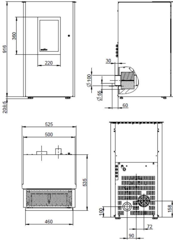
Abb. 102: Maßzeichnung "Pat selection eq" Airplus
