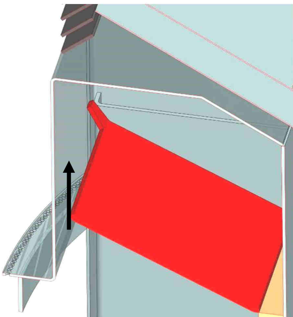
Abb. 58: Durchbrandschlitz Umlenkplatte
