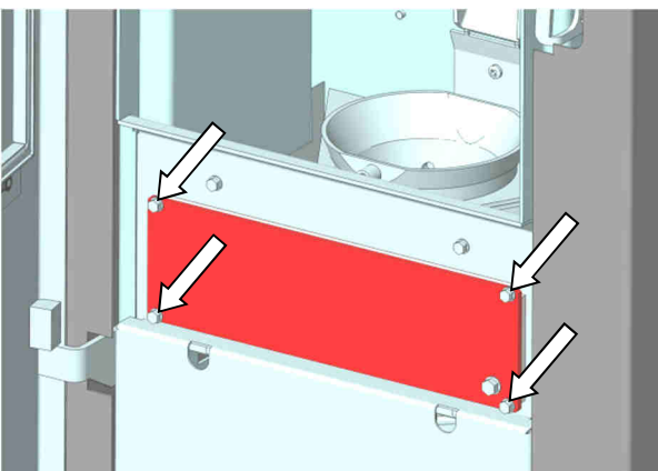
Abb. 79: Demontage Revisionsdeckel
