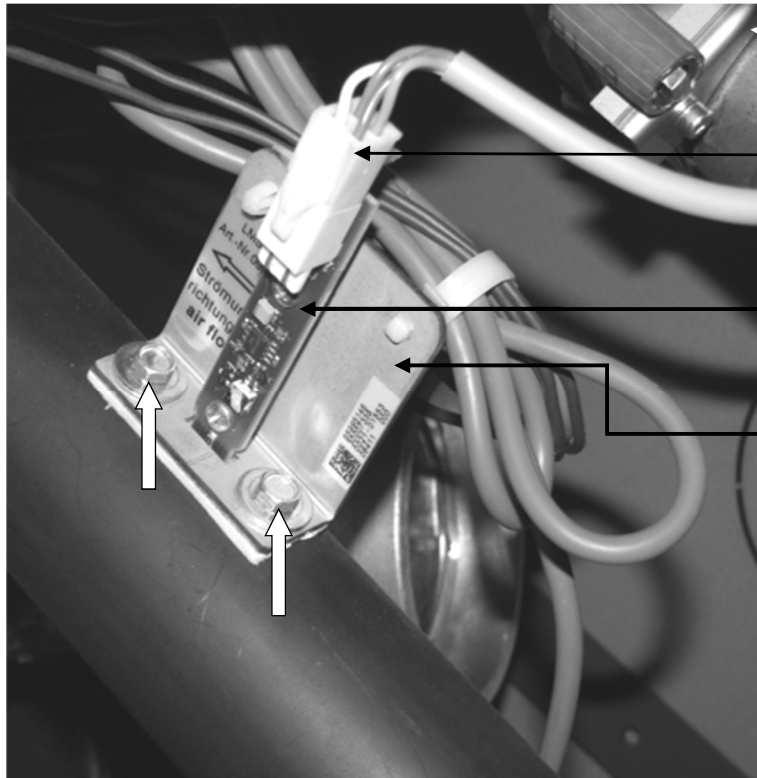
Abb. 94: Luftmengensensor
