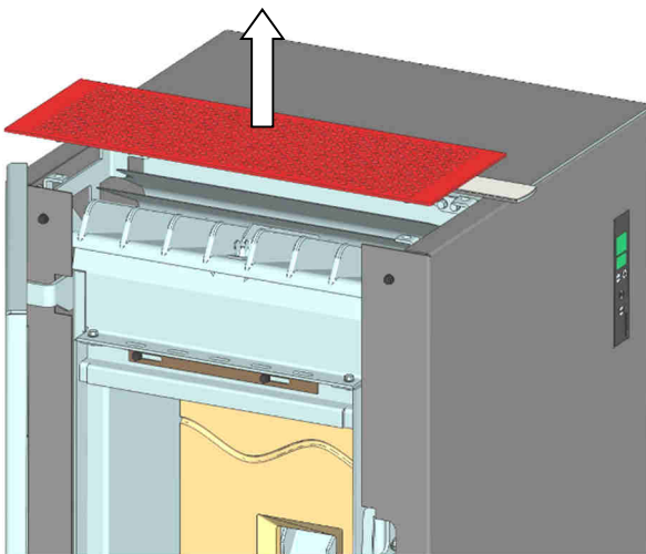
Abb. 37: Entnahme Konvektionsdeckel
