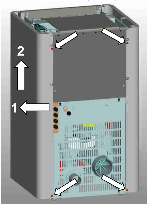
Abb. 44: Schrauben Rückwand Jack/Jack eq
