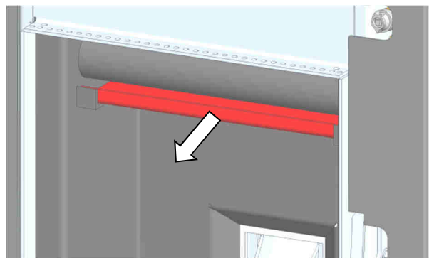
Abb. 76: Entnahme untere Umlenkplatte
