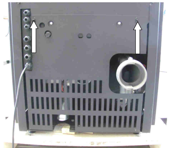
Abb. 93: Demontage hintere Verkleidung Topline New Motion
