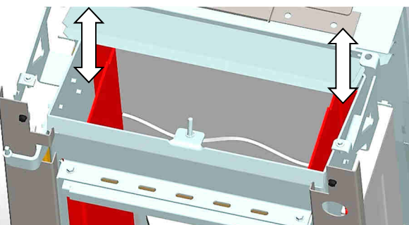
Abb. 49: Reinigung innenliegende Heizgaszüge
