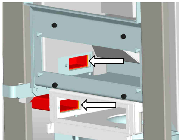
Abb. 55: Reinigung Heizgaszüge unten
