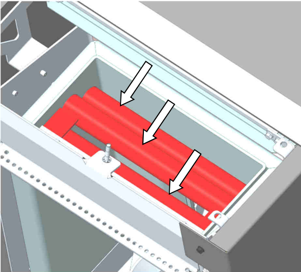
Abb. 78: Reinigung Wasserwärmetauscher
