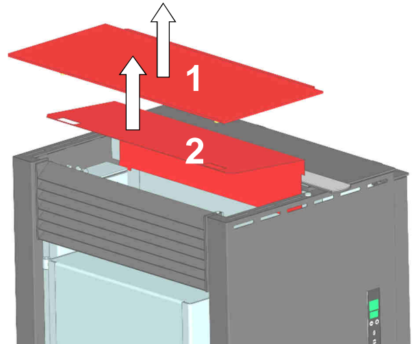
Abb. 59: Demontage Deckel und oberes Strahlungsschutzblech
