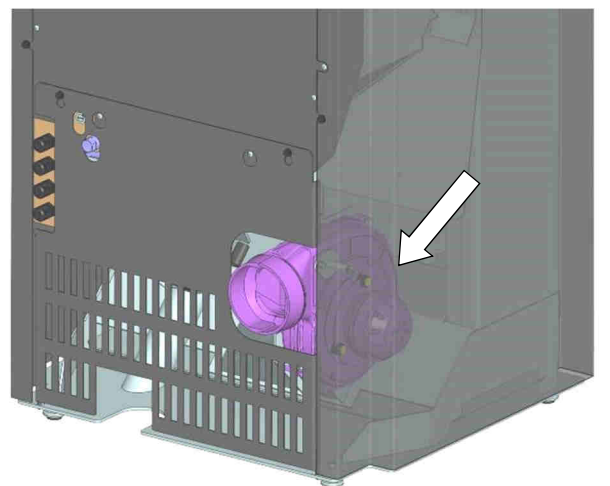
Abb. 72: Position Rauchgasgebläse
