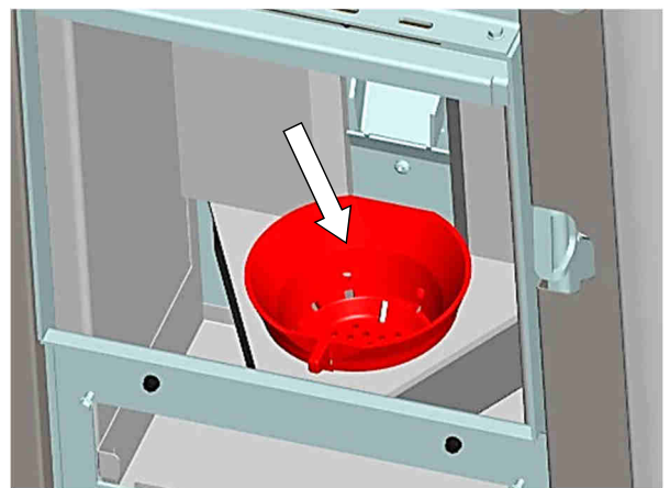
Abb. 51: Reinigung Brennertopf
