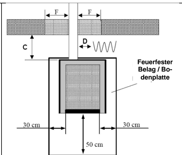
Abb. 96: Beispiel mit Verbindungsstück durch Wand mit brennbaren Bauteilen zum Schornstein
