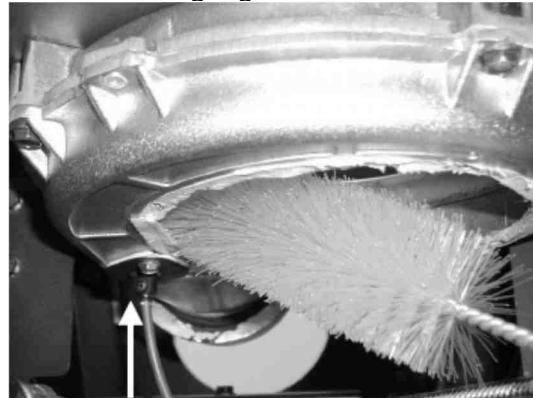
Abb. 88: Position Rauchgasfühler
