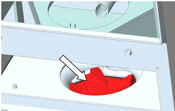
Abb. 84: Flügelrad Rauchgasgebläse
