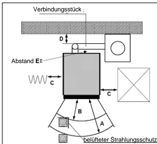
Abb. 95: Beispiel mit Verbindungsstück zum Schornstein innerhalb des Aufstellungsraums
