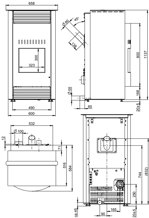
Abb. 104: Maßzeichnung "Topline New Motion" Airplus
