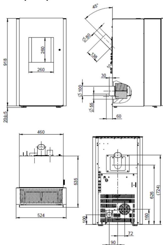
Abb. 98: Maßzeichnung "Frank eq" Airplus
