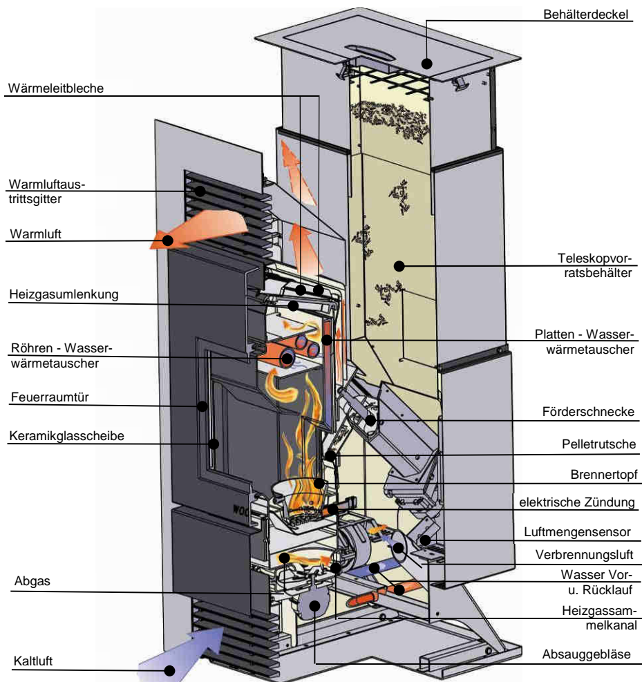
Abb. 4: Funktionsskizze PE Waterplus
