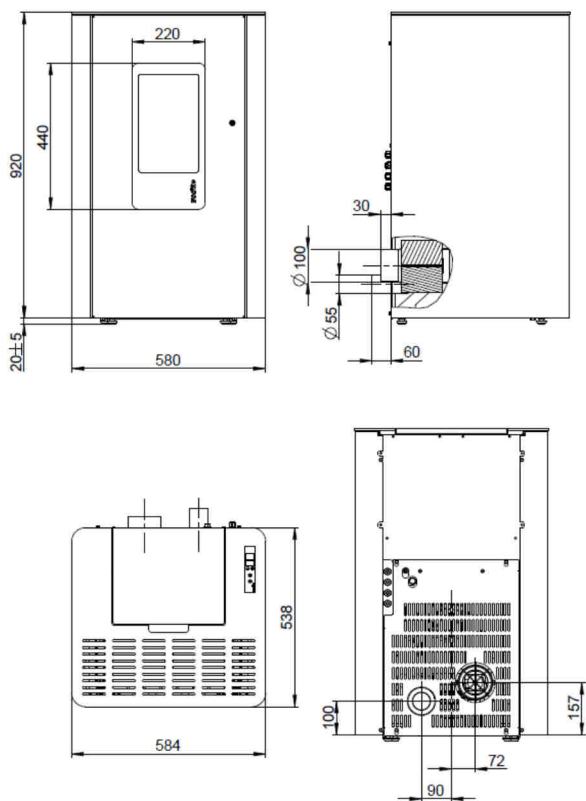
Abb. 100: Maßzeichnung „Jack eq“ Airplus
