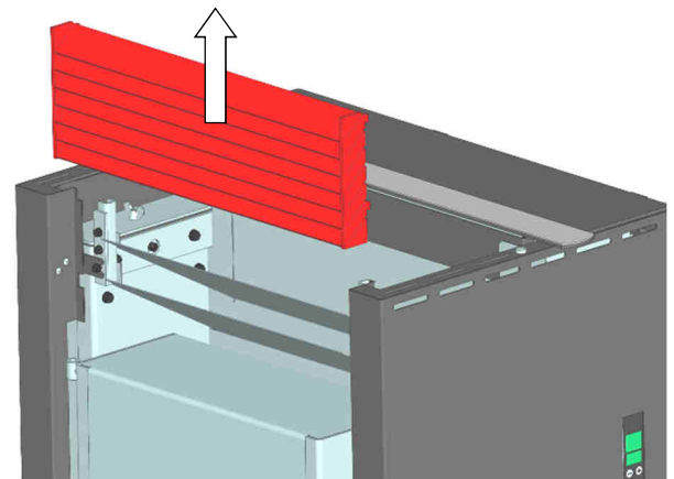
Abb. 60: Demontage Konvektionsgitter
