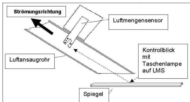
Abb. 90: Funktionsskizze Luftmengensensor
