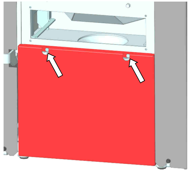
Abb. 85: Demontage Verkleidungsschürze
