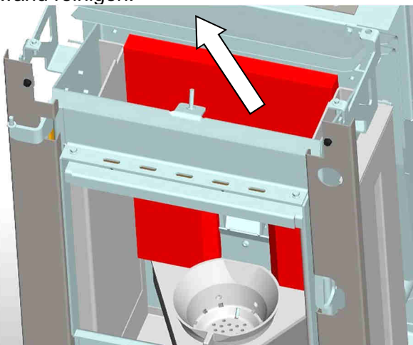
Abb. 48: Entnahme Schamotte
