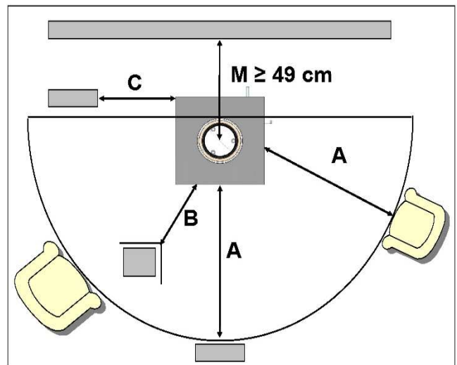
Abb. 3: Brandschutzabstände Ofen gerade
