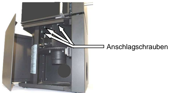
Abb. 7: Position Anschlagsschrauben
