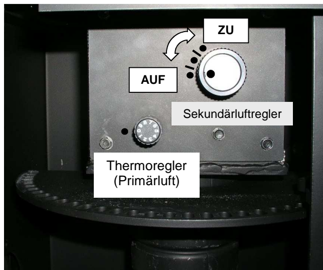
Abb. 26: Einstellung Thermoregler und Sekundärluftregler
