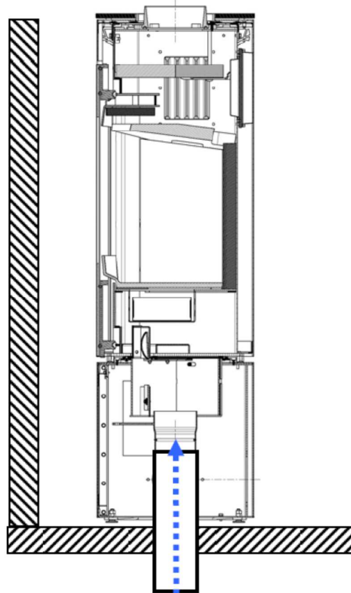
Abb. 16: Von unten Keller / UG (Empfehlung)
