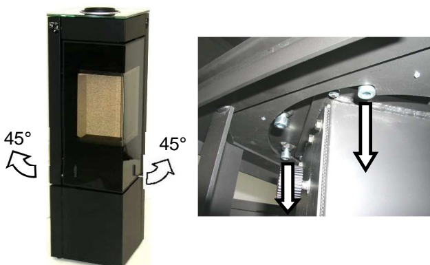
Abb. 8: Schwenkbereich \pm 45^\circ nach links und rechts
