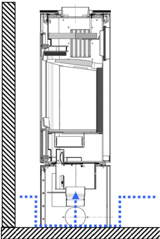
Abb. 15: Ansaugung aus dem Aufstellraum
