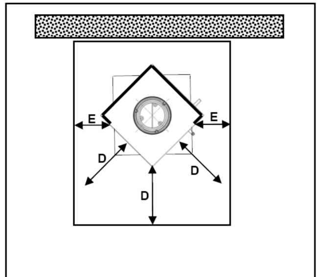
Abb. 6: Funkenschutzvorlage – Ofen gedreht
