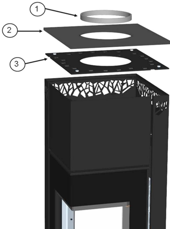
Abb. 11: Entfernen oberer Deckel (nur KK95-1)
