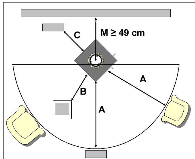
Abb. 4: Brandschutzabstände Ofen gedreht
