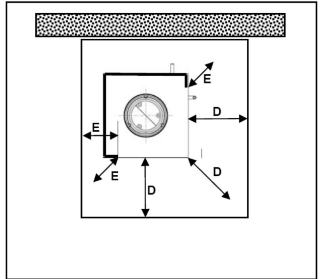
Abb. 5: Funkenschutzvorlage – Ofen gerade
