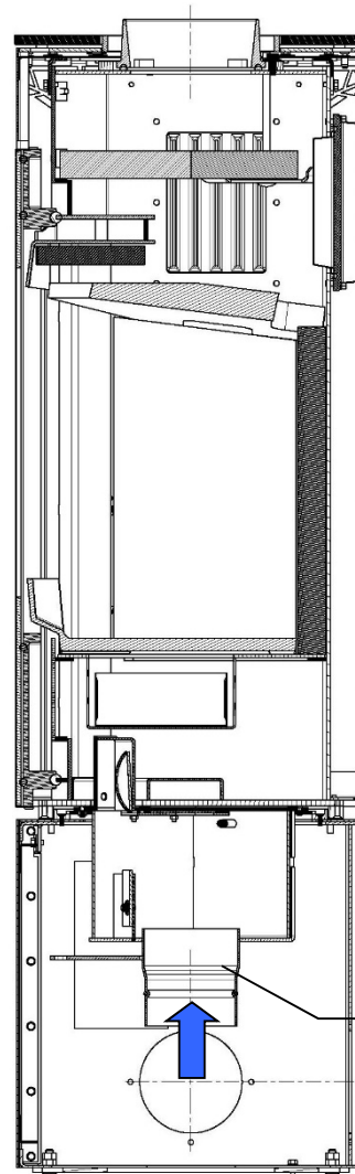
Abb. 14: Zentraler Verbrennungsluftstutzen (Schnittbild)
