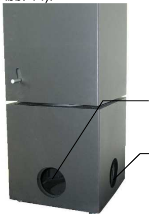
Abb. 13: Sockel mit Ansaugöffnungen und Anschlussöffnung für Verbrennungsluftleitung
