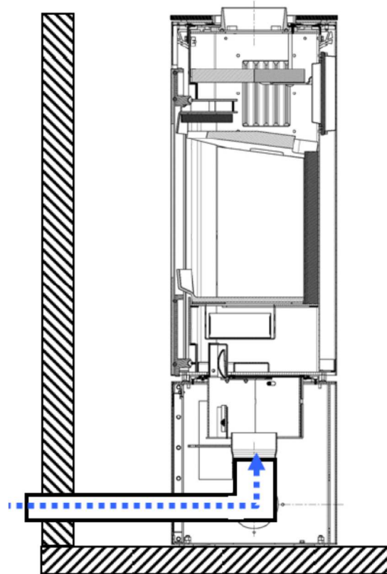
Abb. 17: Vom Nebenraum oder über separaten Luftschacht
