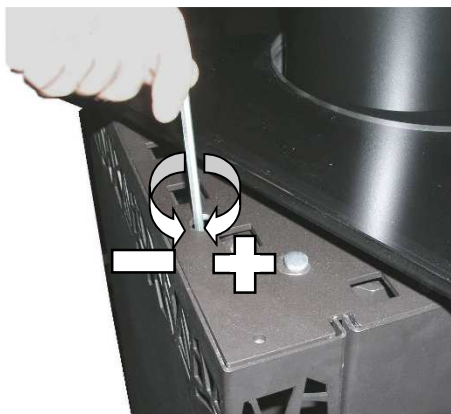
Abb. 21: Einstellen Türvorspannung
