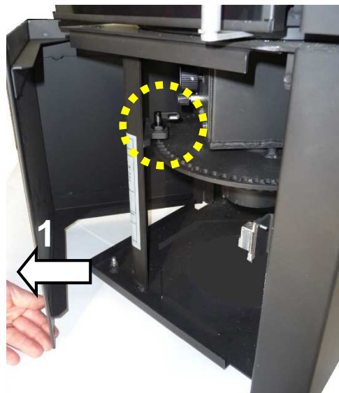
Abb. 22: Position Arretierungshebel
