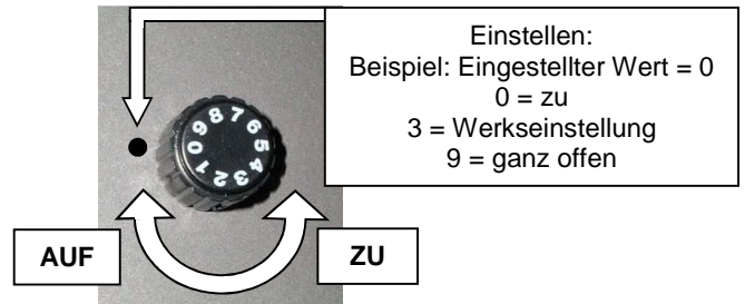
Abb. 27: Einstellung Thermoregler
