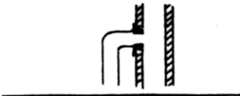
Falschluff durch undichten Rohranschluß
