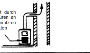
Falschluff durch offenen Rohranschluß
